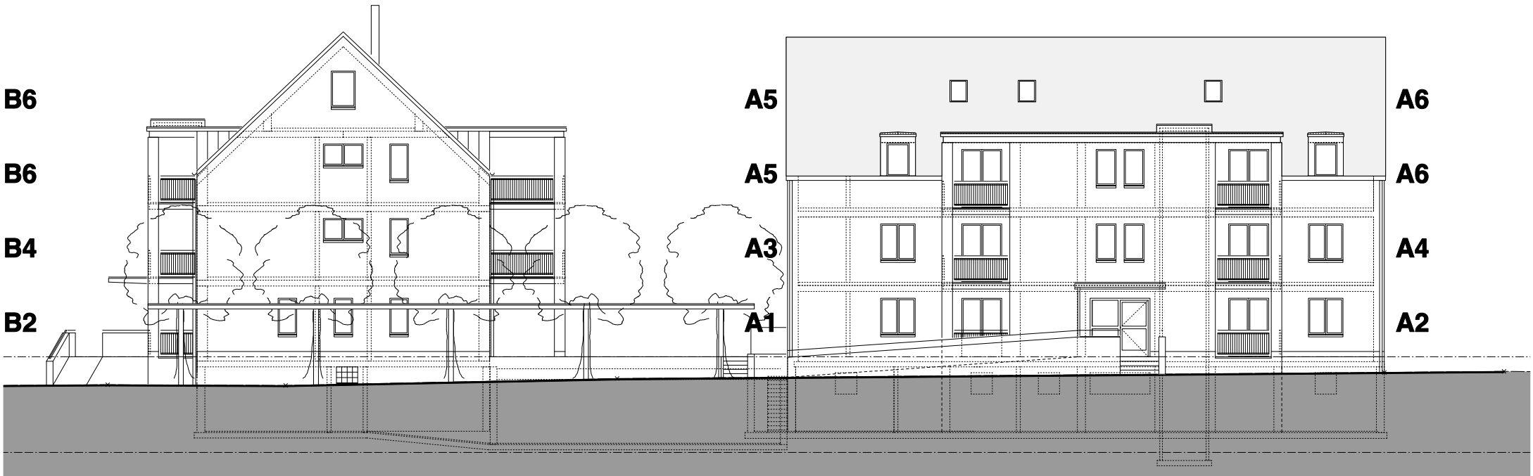
NORDFASSADE
