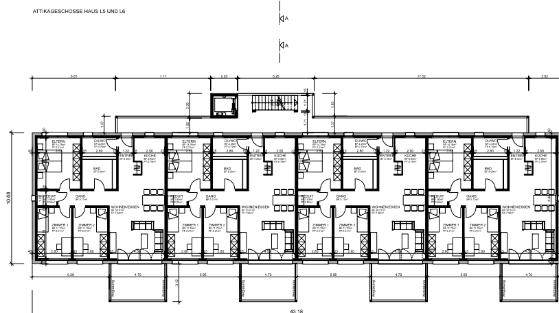
HAUS L5: 1.-3. OBERGESCHOSS / HAUS L6: 1. OBERGESCHOSS
