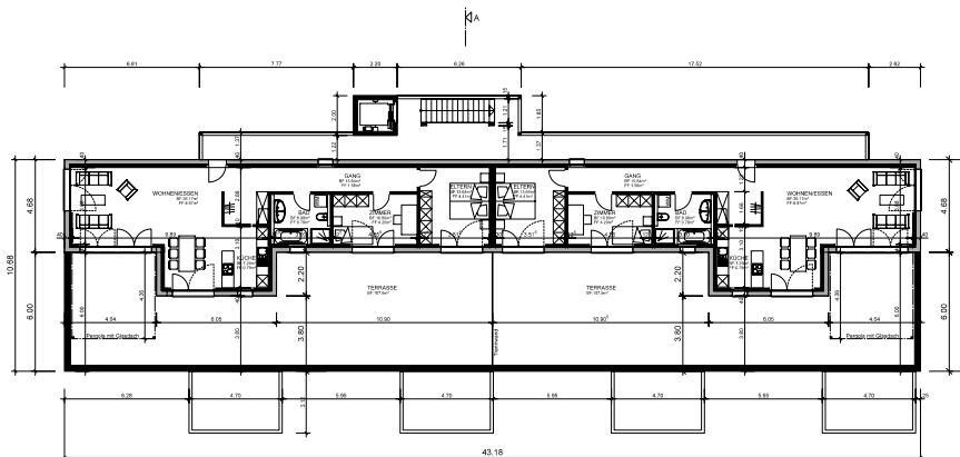
ATTIKAGESCHOSS HAUS L5 UND L6
