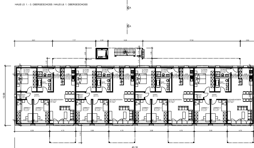
ERDGESCHOSS HAUS L5 UND L6
